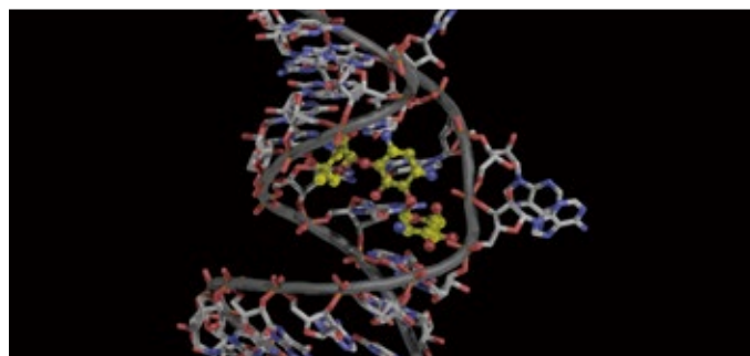
当研究室で解析したRNA-医薬品複合体の立体構造 Three-dimensional structure of RNA-drug complex analyzed in our laboratory.
